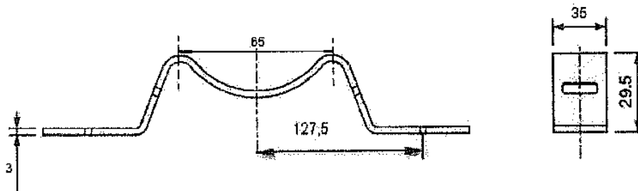
Приложение №3: Монтажни планки за монтаж на стълб.
