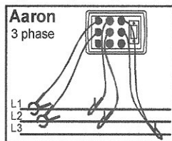
3-фазна, 3-проводна схема с 2 токови клещи
