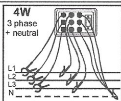
3-фазна, 4-проводна схема
